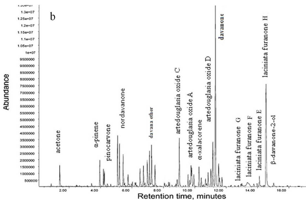
شکل ۱: طیف‌های کروماتوگرام حاصل از آنالیز اسانس گیاه A. persica به دو روش استخراج با تقطیر (a) و سیال فوق بحرانی GC/MS با دستگاه (b)
