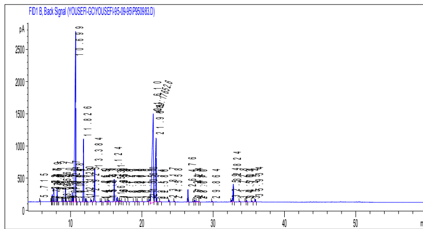
شکل ۴: کروماتوگرام GC اسانس مرزه بختیاری از جمعیت سپیدان
