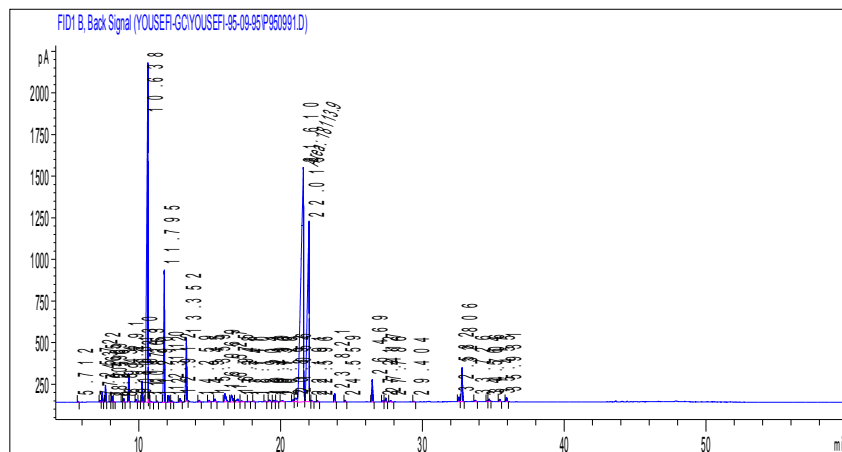
شکل ۵: کروماتوگرام GC اسانس مرزه بختیاری از جمعیت آباه-انارک
