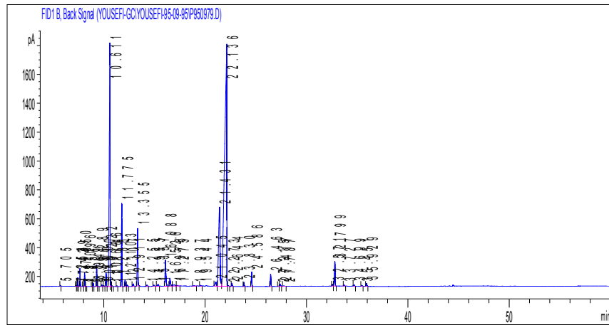
شکل ۳: کروماتوگرام GC اسانس مرزه بختیاری از جمعیت آباه- دیدگان
